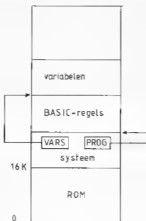
Afb. 7-1 Indeling van het BASIC-geheugen
